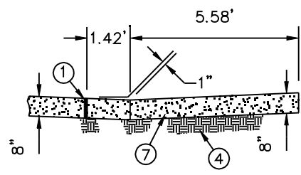
SEC. A-A
